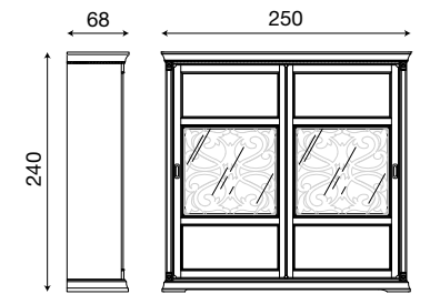
L. 250 P. 68 H. 240
