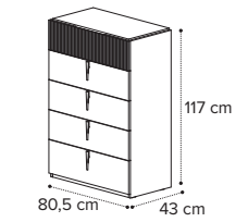
Settimino Tallboy Комод 5 ящ.
